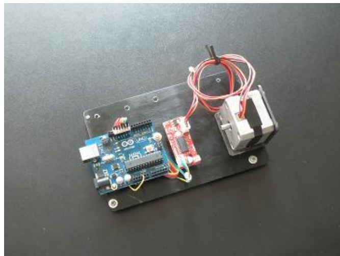
ARDUINO uno + EasyDriver + Step motor
